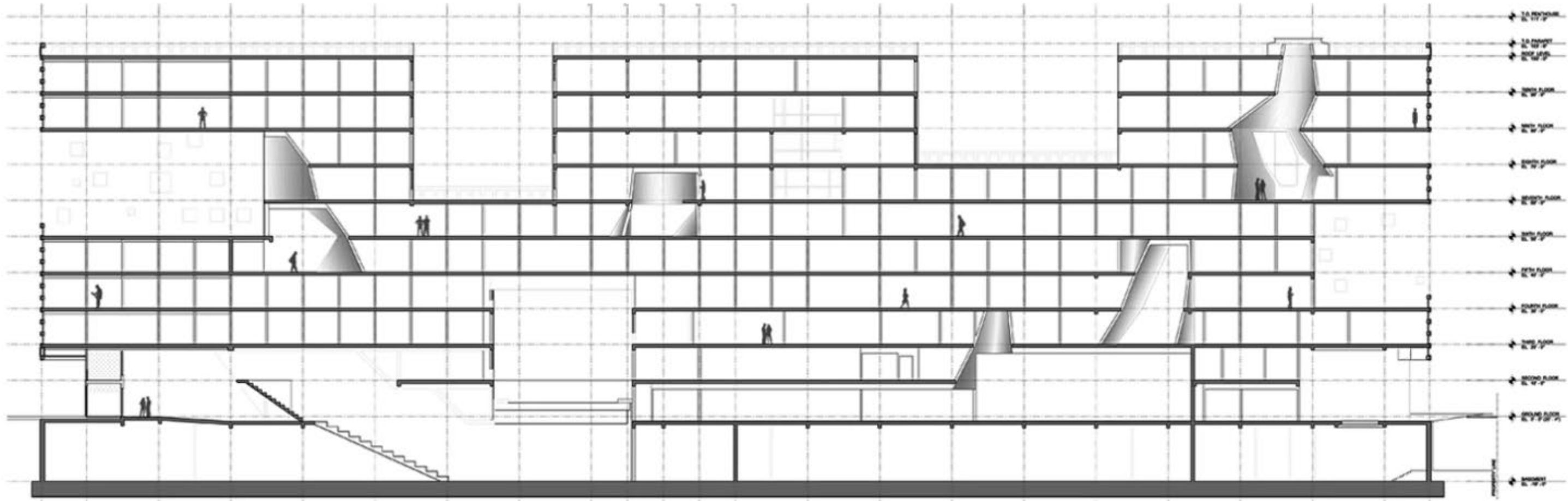
1 LONGITUDINAL SECTION 3-132'-1-0"
