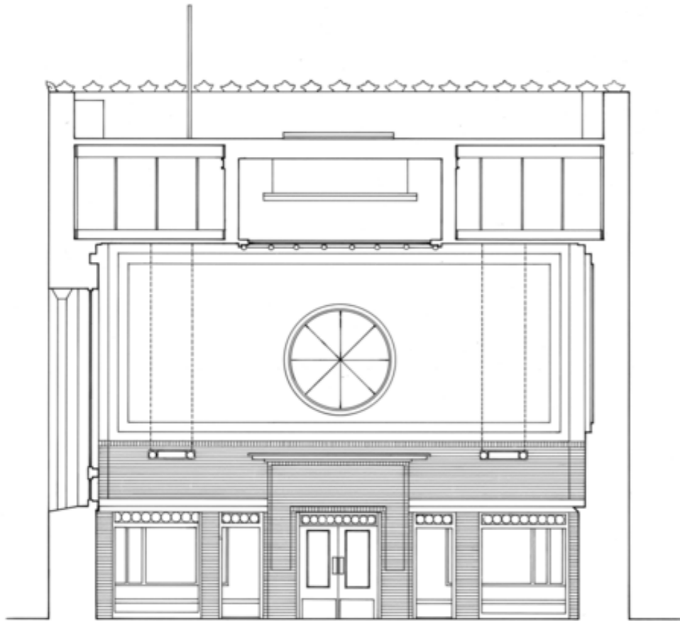
SECTION D-D
