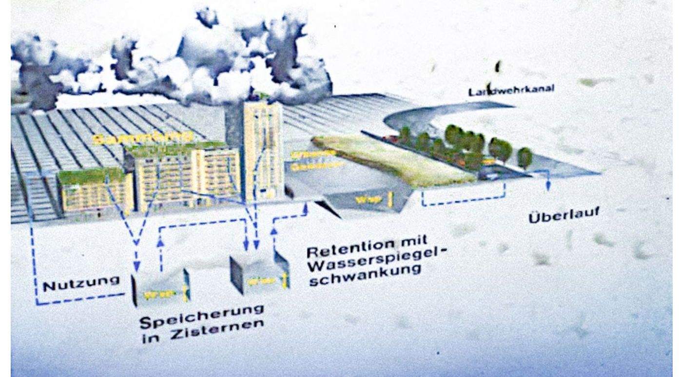
Berlin Potsdamer Platz Regenwassermanagement
