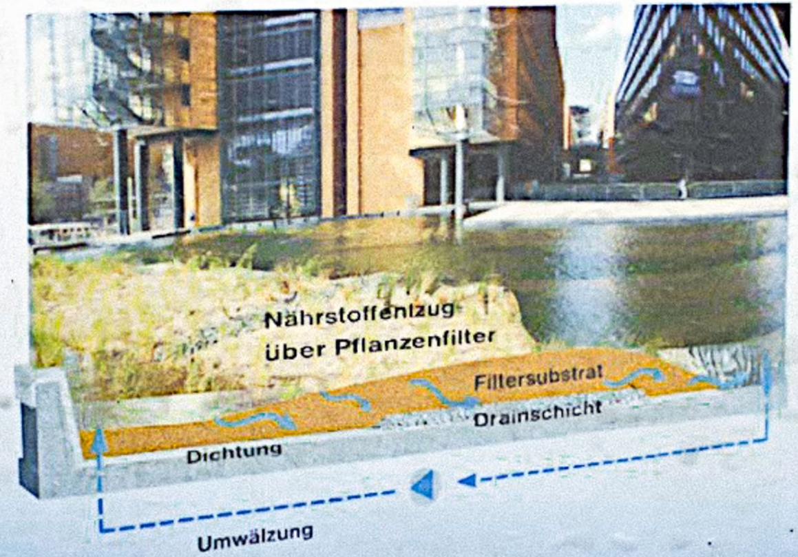
Berlin Potsdamer Platz Reinigungsbiotop
