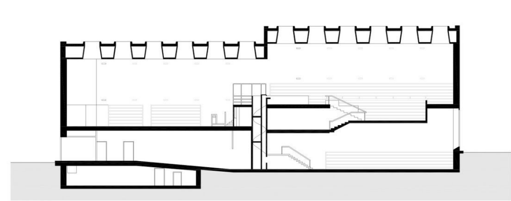
Sección a-a'
