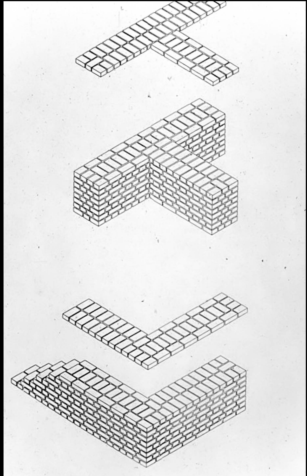
Lange House | Mies van der Rohe | Krefeld, Germany | 1923
